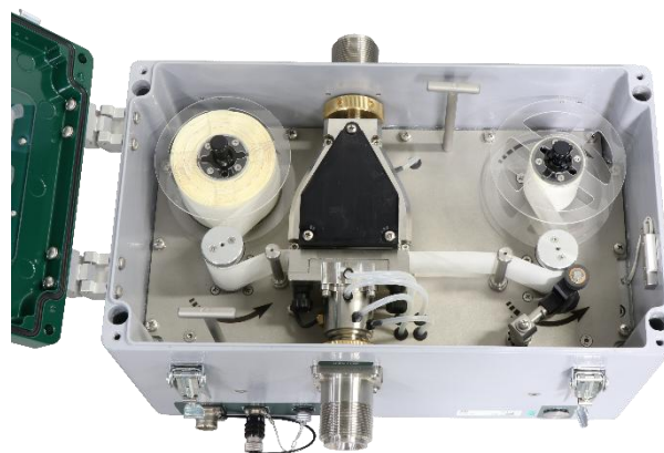
Otevřená skříň detektoru CPD-13
